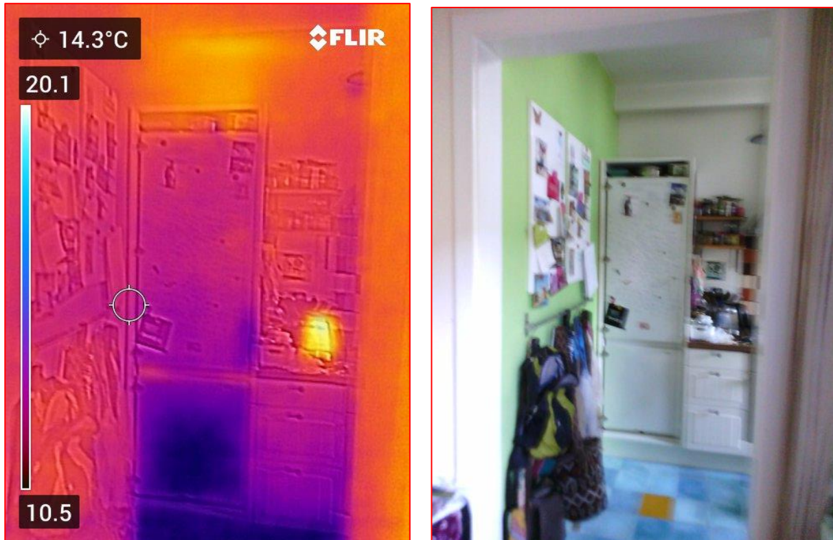
Figuren 1. Op deze Infra-Rood (IR) foto is te zien dat de koelkast uit twee delen bestaat met aan de onderzijde de diepvries. De temperatuurschaal staat links langs de foto. De thermische isolatie van de diepvries (onder de koelkast) laat te wensen over. Waarschijnlijk is dit een oude koelkast. De warme lucht die boven achter de koelkast uit komt verwarmt het plafond.
