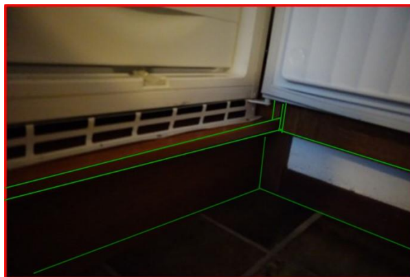
Figuren 8. Links . Bestaand. Rechts . Door een strook uit de voorkant bodem van de keukenkast te zagen (eenvoudig) wordt er een opening van >200 cm 2 gemaakt en kan de ventilatielucht er langs de plint van onderen achter de deur langs omhoog en dan door het rooster onder langs en achter de koelkast naar boven.
